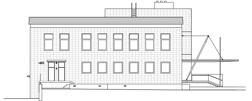
ZÁPADNÍ A VÝCHODNÍ POHLED / WEST AND EAST
