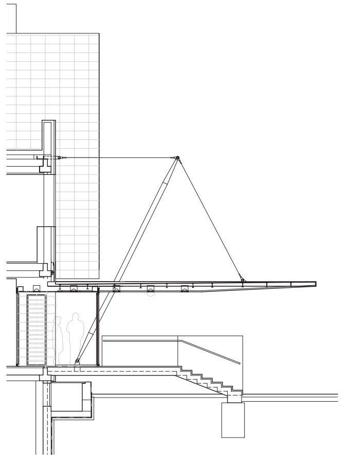
ŘEZ HLAVNÍM VSTUPEM / MAIN ENTRANCE SECTION
